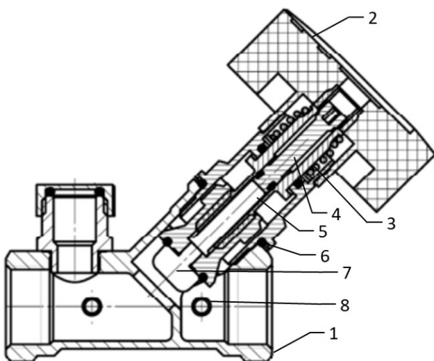
Рис 1. Основные элементы конструкции.
